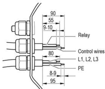
Abb. 1: Empfohlene Abmantellängden in mm (innerhalb Klemmkasten)
