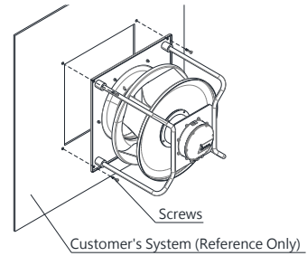
带框风扇
