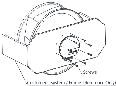
单体风扇
