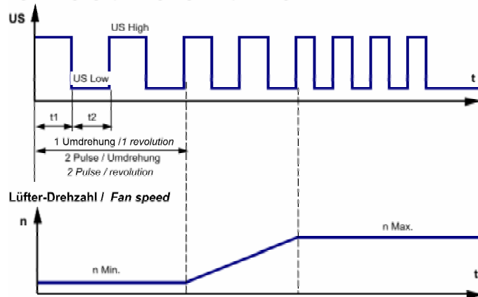
Signal-Ausgangsspannung / Signal output voltage
